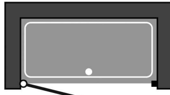
1 Açılır Menteşeli Kapı
