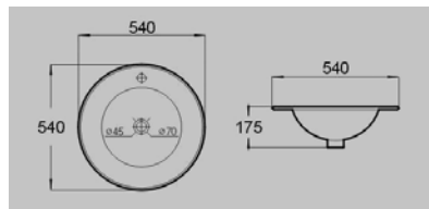
1 E-3050A 540x540x175 mm Yarım tezgah üstü lavabo Semi-counter basin
